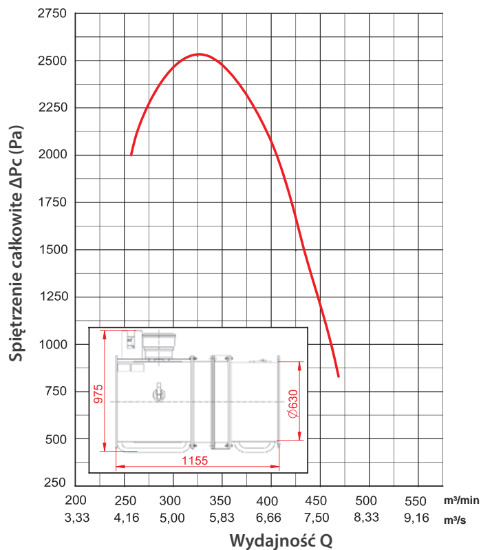
Charakterystyka wentylatora GWE-630B/18,5
