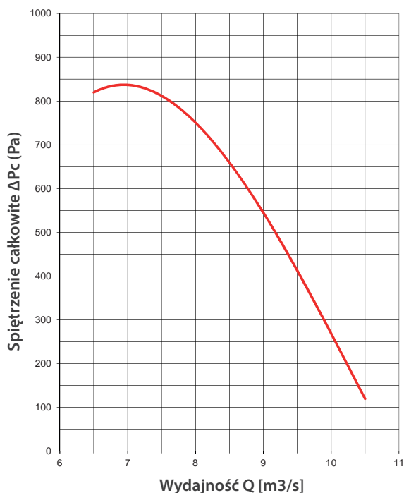
Charakterystyka wentylatora WLE-800E/1
